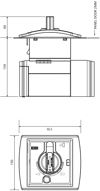
Panel Door Cutout
